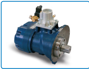
Gruppo vite con valvola di aspirazione.
